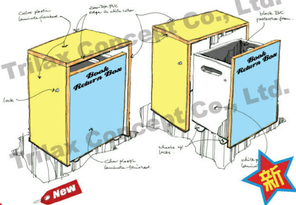
tommy 還書車 - Book Return Box 尺寸 (Size) - 600mm(W) x 900mm(H) x 500mm(D)
